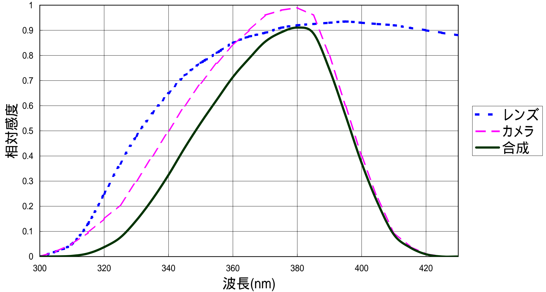
分光感度特性(参考値)
